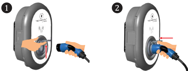
Abb. 1: TECHNIVOLT 100
