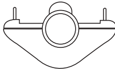
Natürliche Wellen
